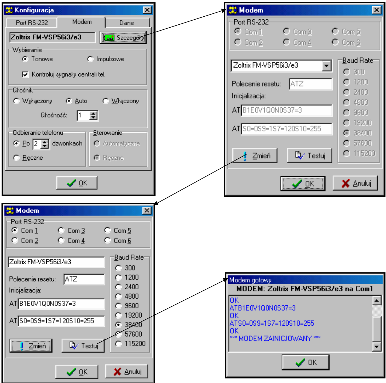
Rysunek 11. Okna dialogowe programu DLOAD10.
