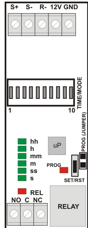
Rysunek 1: Rysunek poglądowy płytki.
